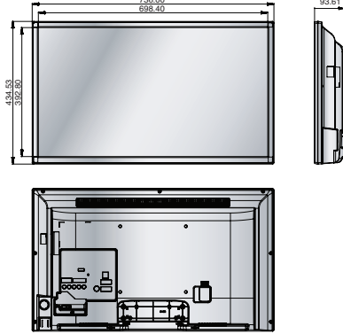
SMT-3230
