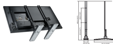
SBM-320ST Ayaklıklık
